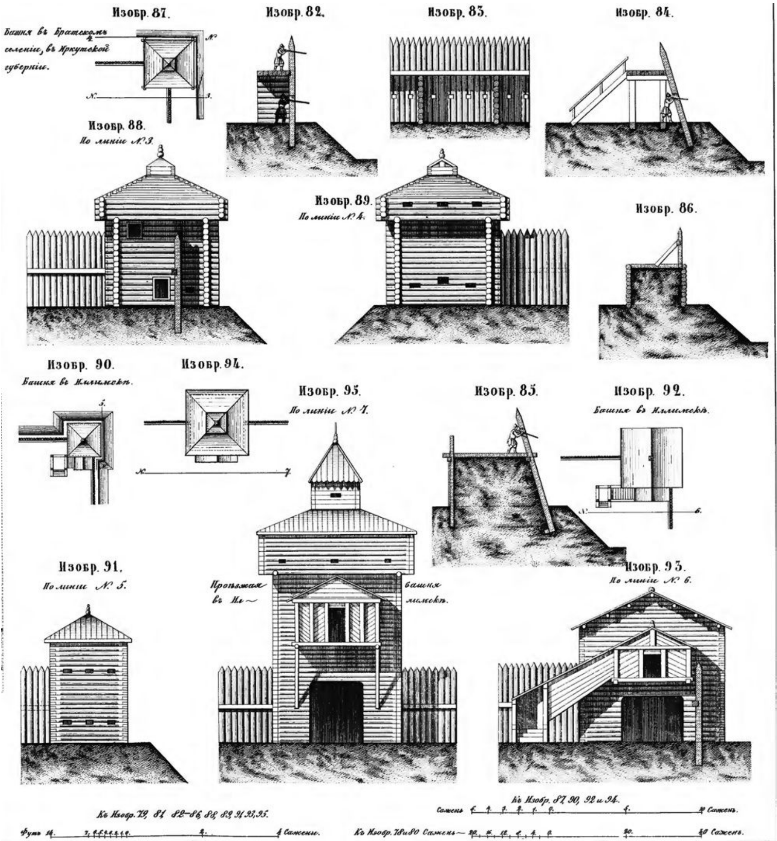
Рис. 4 Реконструкция укреплений по Ф.Ф. Ласковскому
