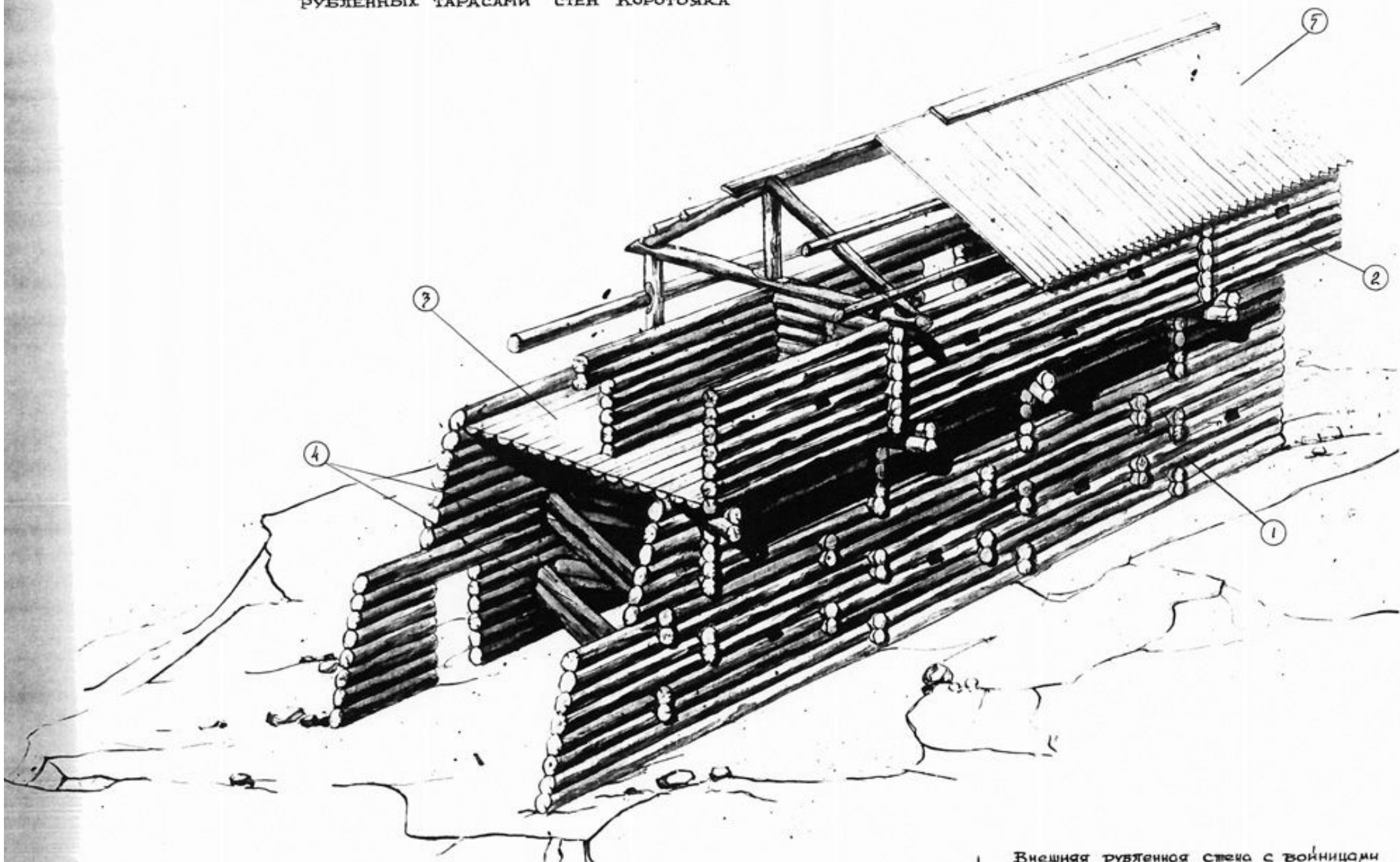
Рис. 2 Конструктивная схема рубленных тарасами стен по Г.А. Каримову
