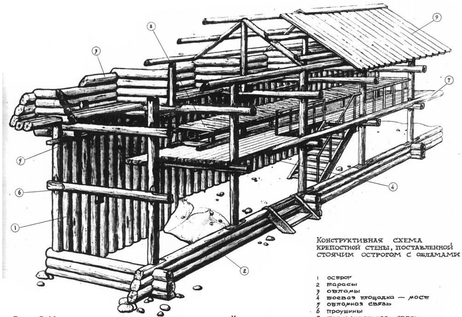
Рис. 3 Конструктивная схема крепостной стены, поставленной стоячим острогом с обламами по Г.А. Каримову
