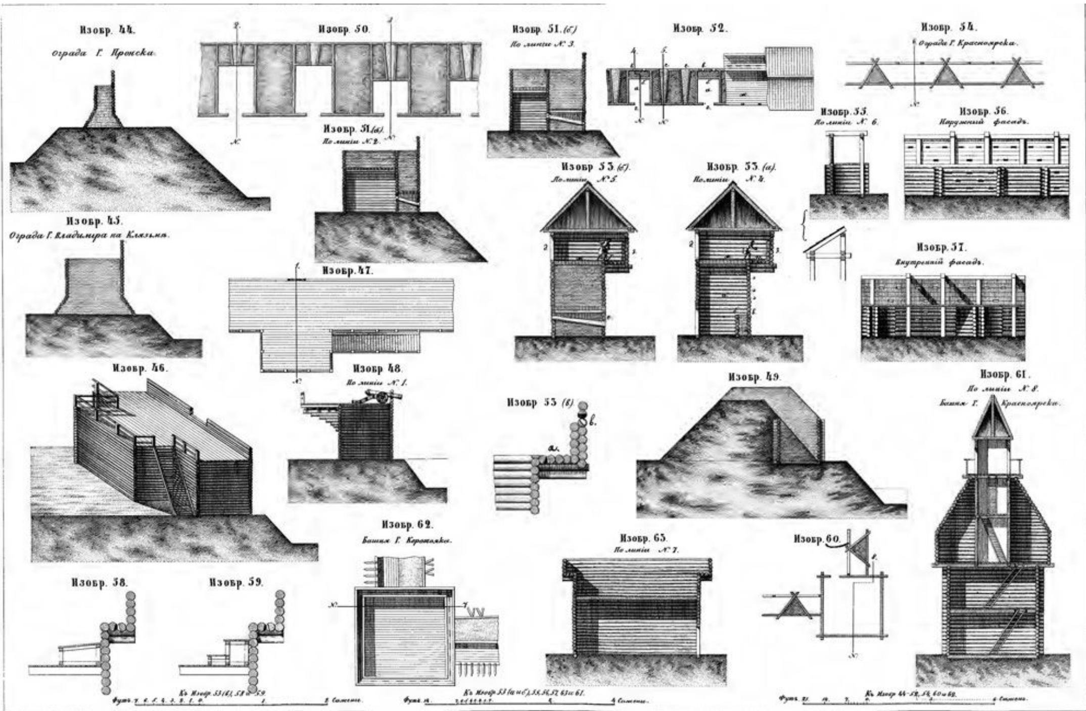
Рис. 5 Реконструкция укреплений по Ф.Ф. Ласковскому
