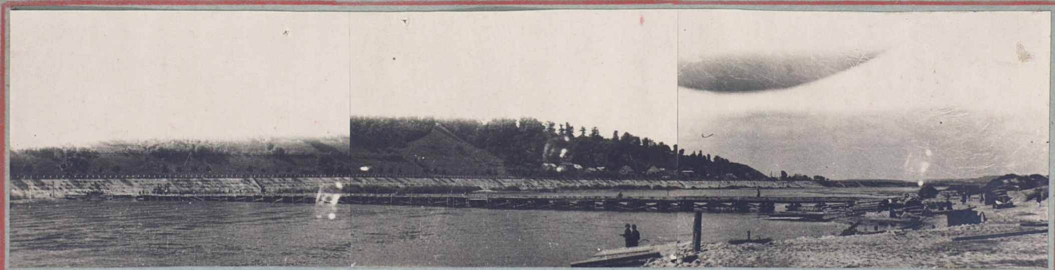
Мост через р. Неман. Грузоподъемность 70 т., построенный 5-м турм. Инж. С. П. Бр.
