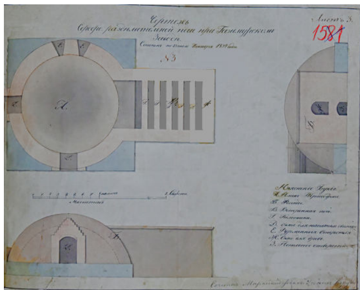
Рис. 2. Чертеж серебряноразделительной печи в Газимурском Заводе 1834 г. [7]
